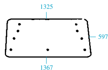
23/4071-17 (D9018, 5130388) Trasero - 9 agujeros Rear - 9 holes
