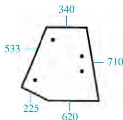
23/4066-3 (D9012, 5124412) Lateral (drcha o izq.) 4 agujeros Side (LH-RH) 4 holes
