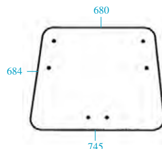
23/4072-73 (D9042, 5136410) Trasero (superior) 6 agujeros Upper rear - 6 holes
