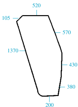
23/4038-4 (D9007, 5124414) Puerta izq. LH door
