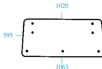
23/4071-12 (D9013, 5108627) Trasero - 7 agujeros Rear - 7 holes
