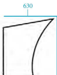
23/4029-5 (D6708, 82002182) Puerta (inf. izq.) Door (Lower LH)
