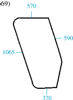
23/4039-3 (D9004, 5108670) Puerta drcha. RH door
