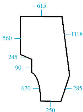
23/4020-27 (D9037, 5136431) Puerta (izq. o drcha) Door (LH-RH)
