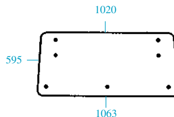
23/4071-13 (D9015, 5113393, 5121385) Trasero - 7 agujeros Rear - 7 holes
