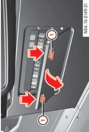
① Стопорные пружины
