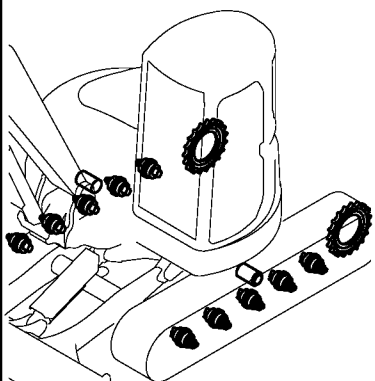
Fig. 16 IDLER & ADJUST
