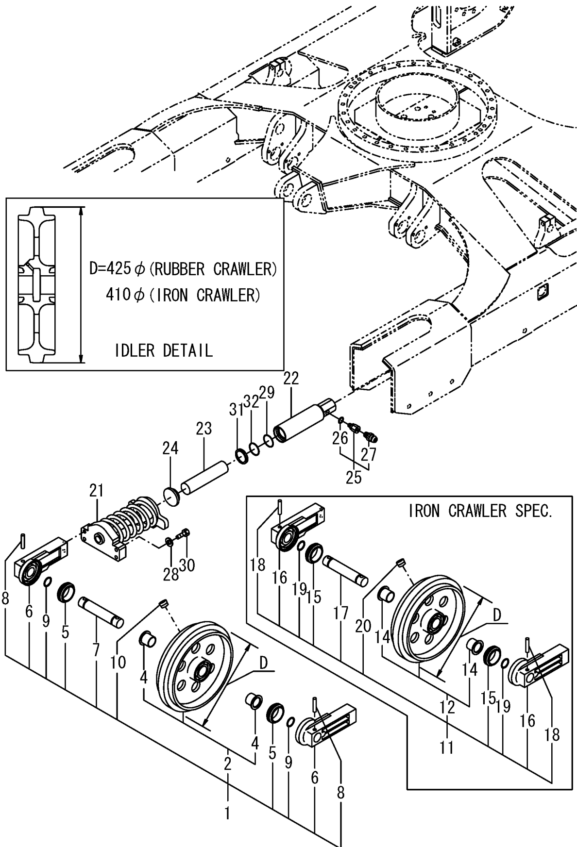
Fig. 16 IDLER & ADJUST
