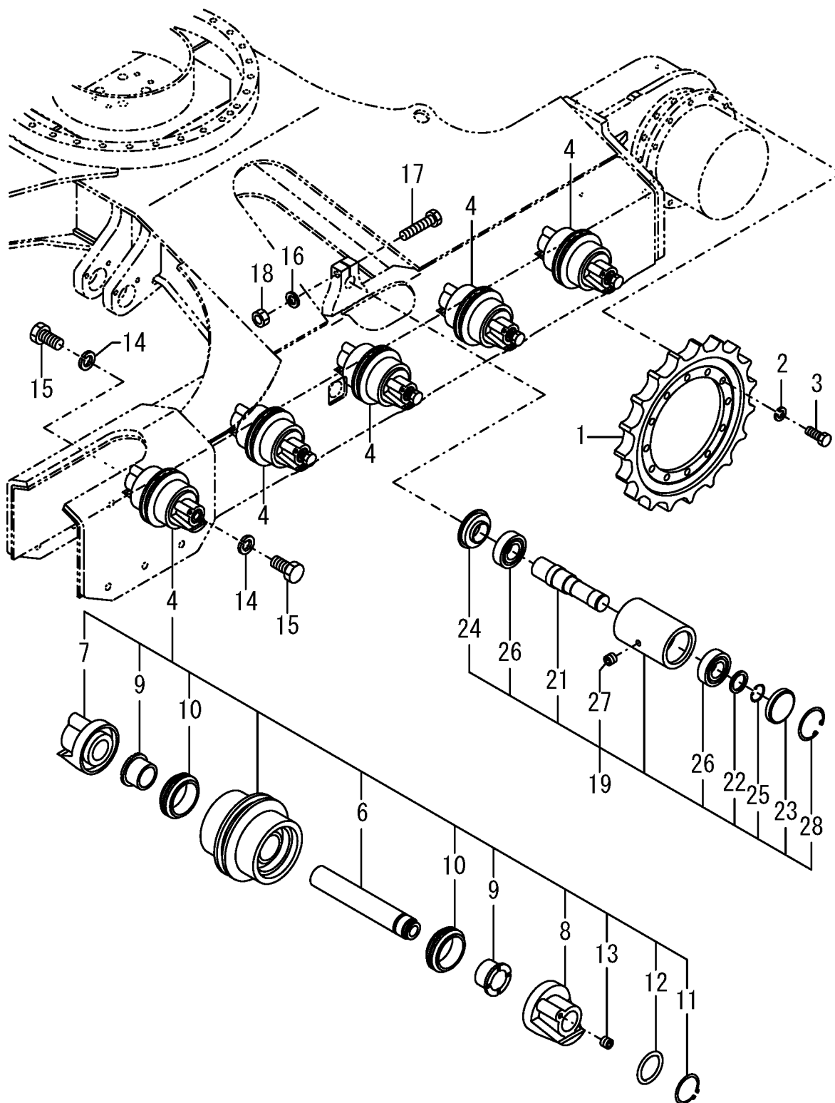
Fig. 15 SPROCKET & ROLLER
