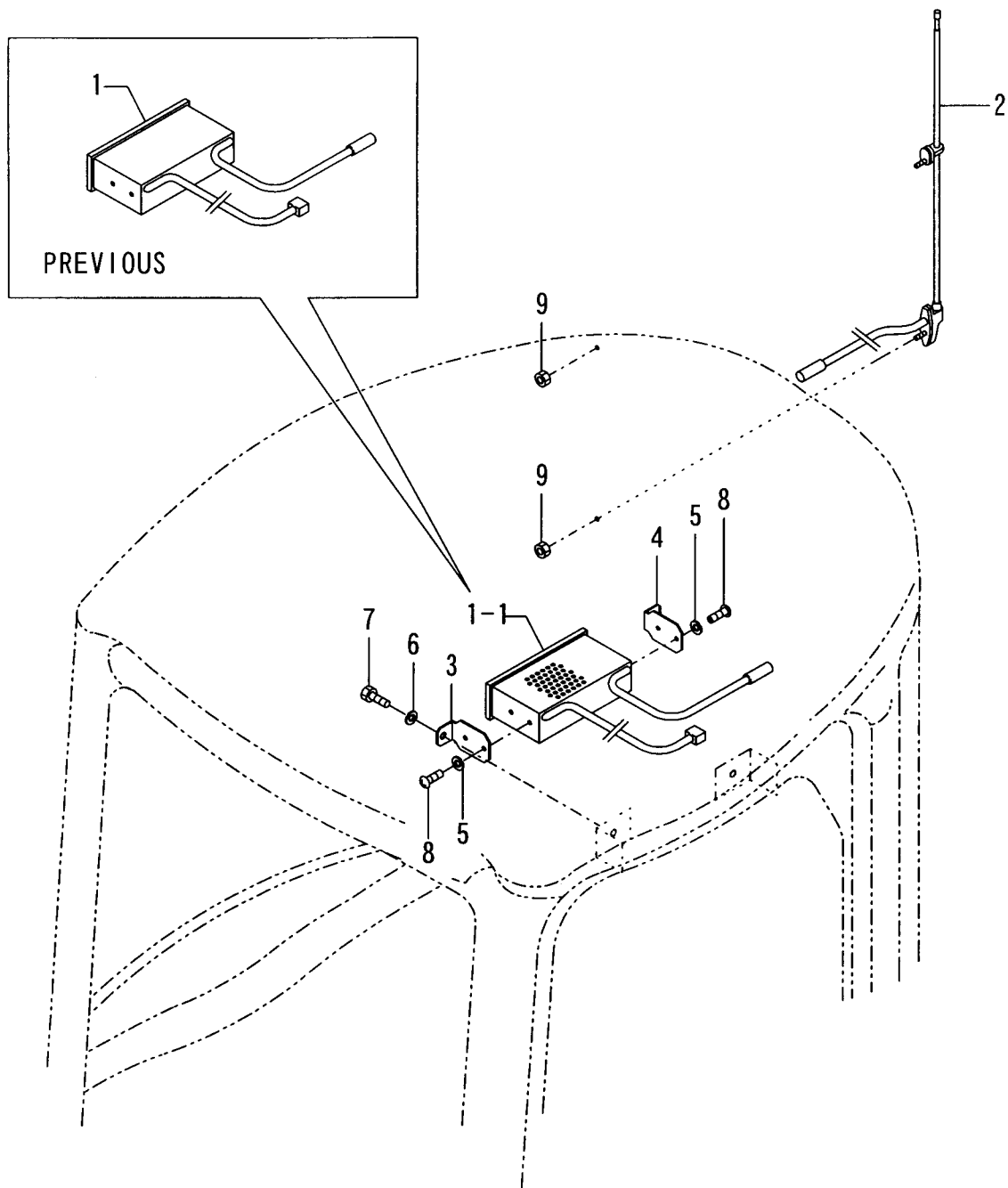
Fig. 14 RADIO
