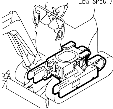
Fig. 27 旋回フレーム TURNING FRAME
