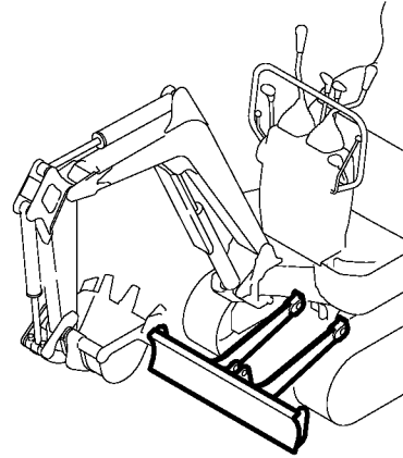
Fig. 70 PTOキット (オプション) P. T. O. KIT (OPTIONAL)
