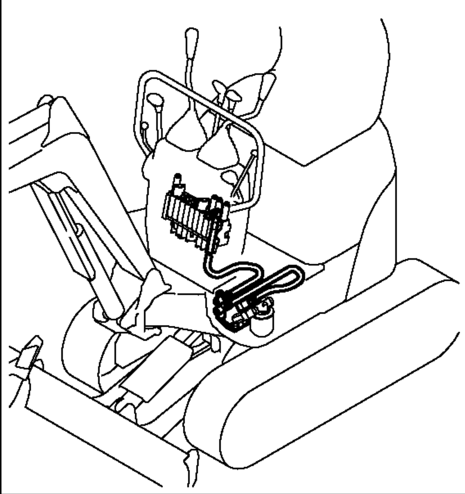
Fig. 57 油圧配管 (PT0フレームント) HYD. OIL PIPING (P. T. O. FREME END)
