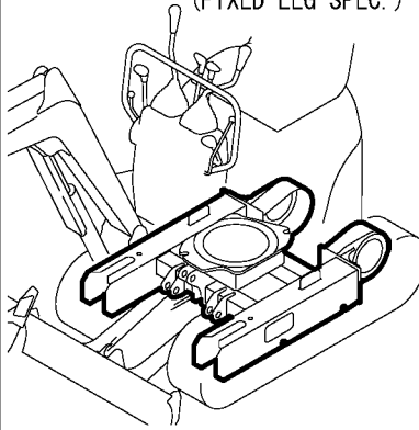
Fig. 26 トラックフレーム (拡張可変脚仕様) TRACK FRAME (WIDEN/SHORTEN VARIABLE LEG SPEC.)
