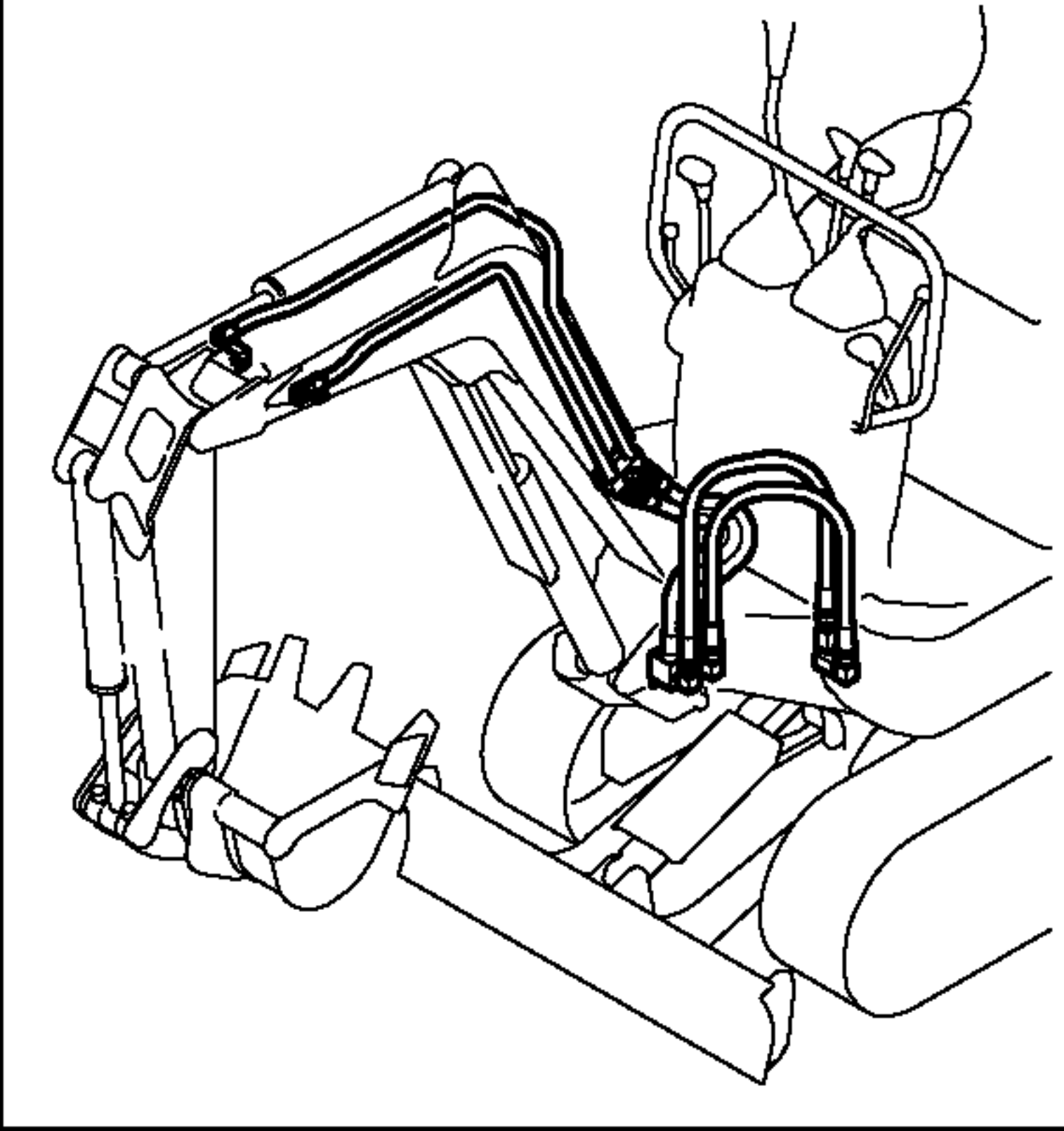
Fig. 62 油圧配管 (PT0ブームント) HYD. OIL PIPING (P. T. O. BOOM END)
