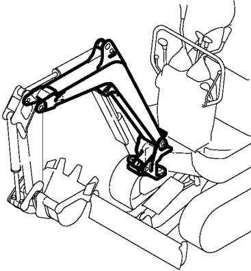
Fig. 64 ブーム & ブームブラケット BOOM & BOOM BRACKET
