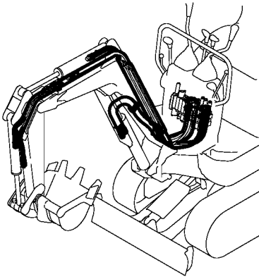
Fig. 62 油圧配管 (PTOブームエンド) HYD. OIL PIPING (P. T. O. BOOM END)
