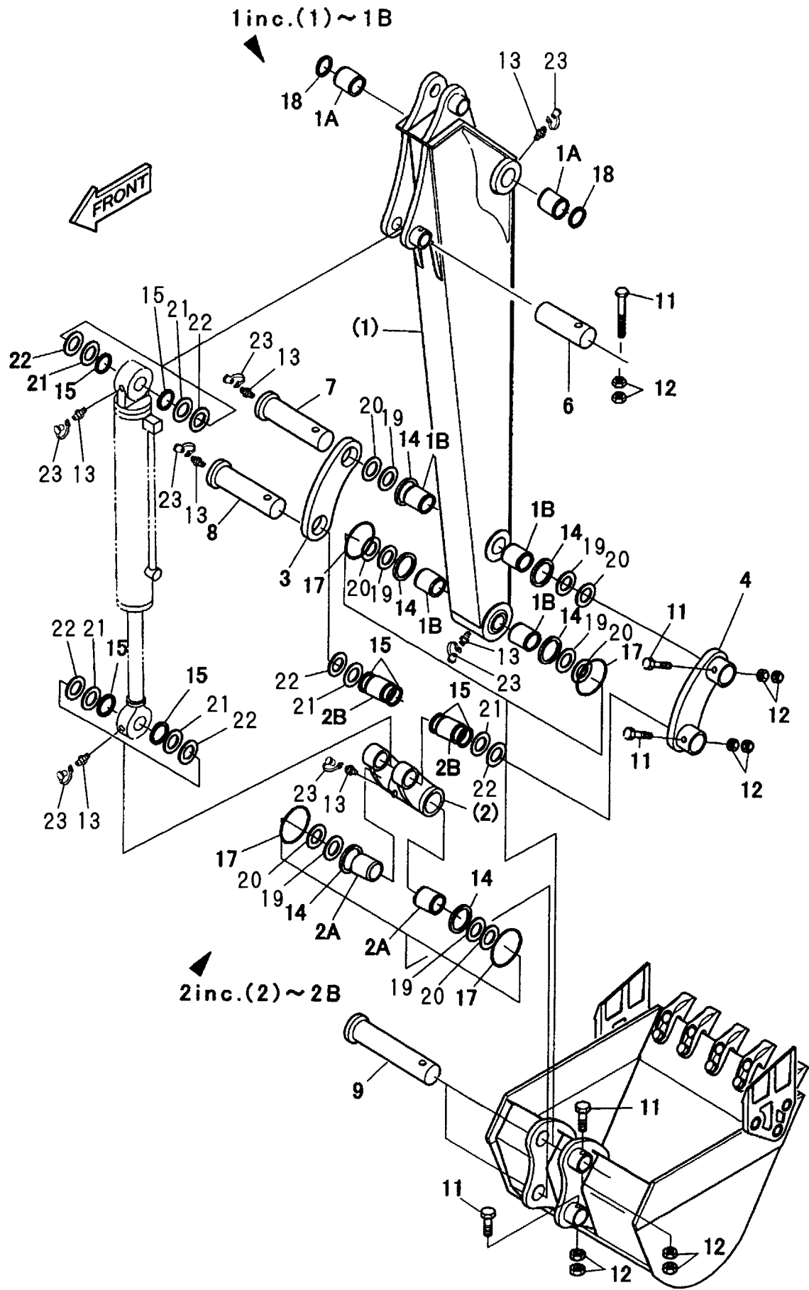
Fig. 140 ARM 1.47M
