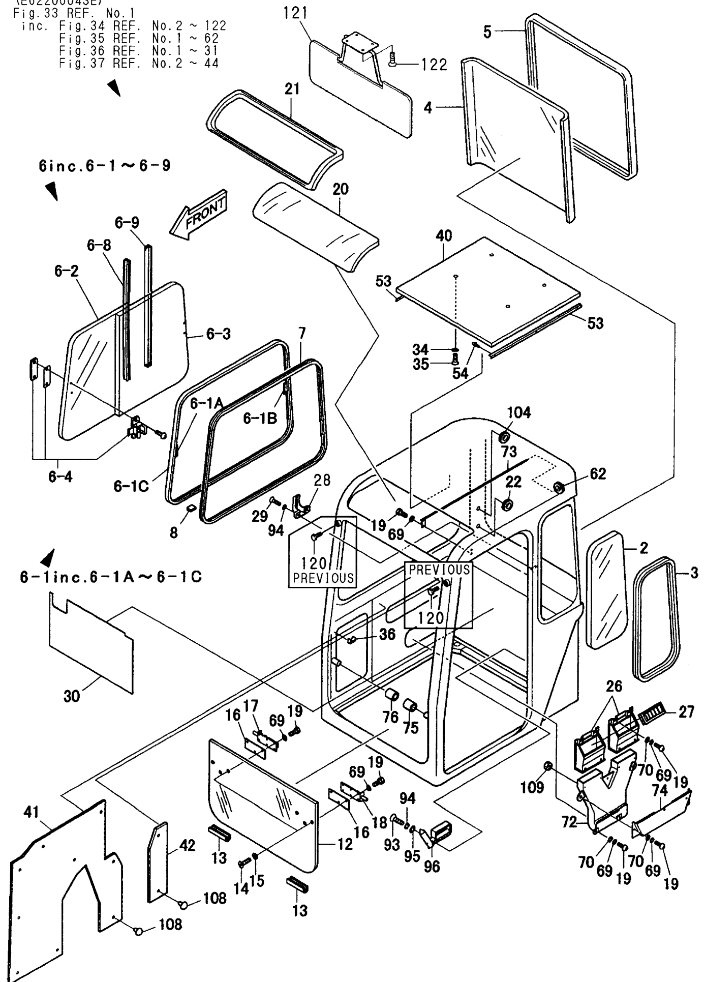
Fig. 34 CABIN (2)
