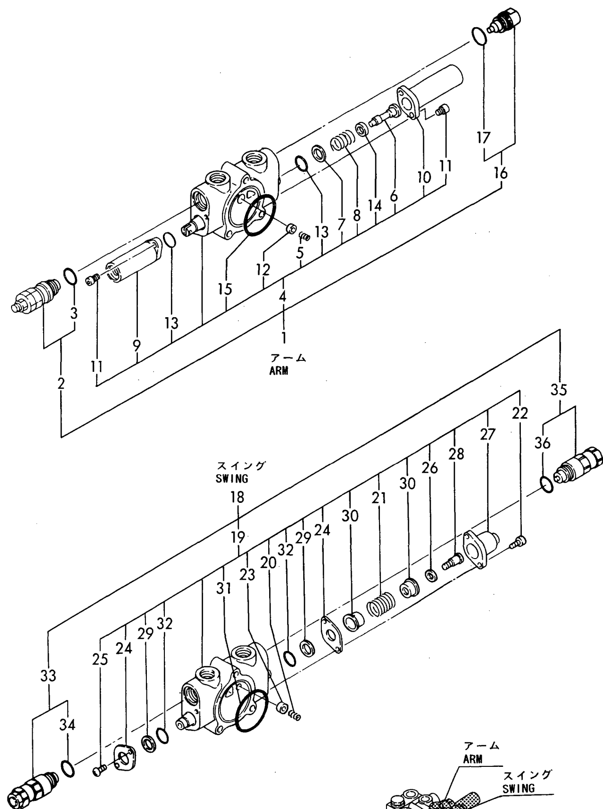
Fig. 42 コントロールバルブ(アーム & スイング) CONTROL VALVE(ARM & SWING)
