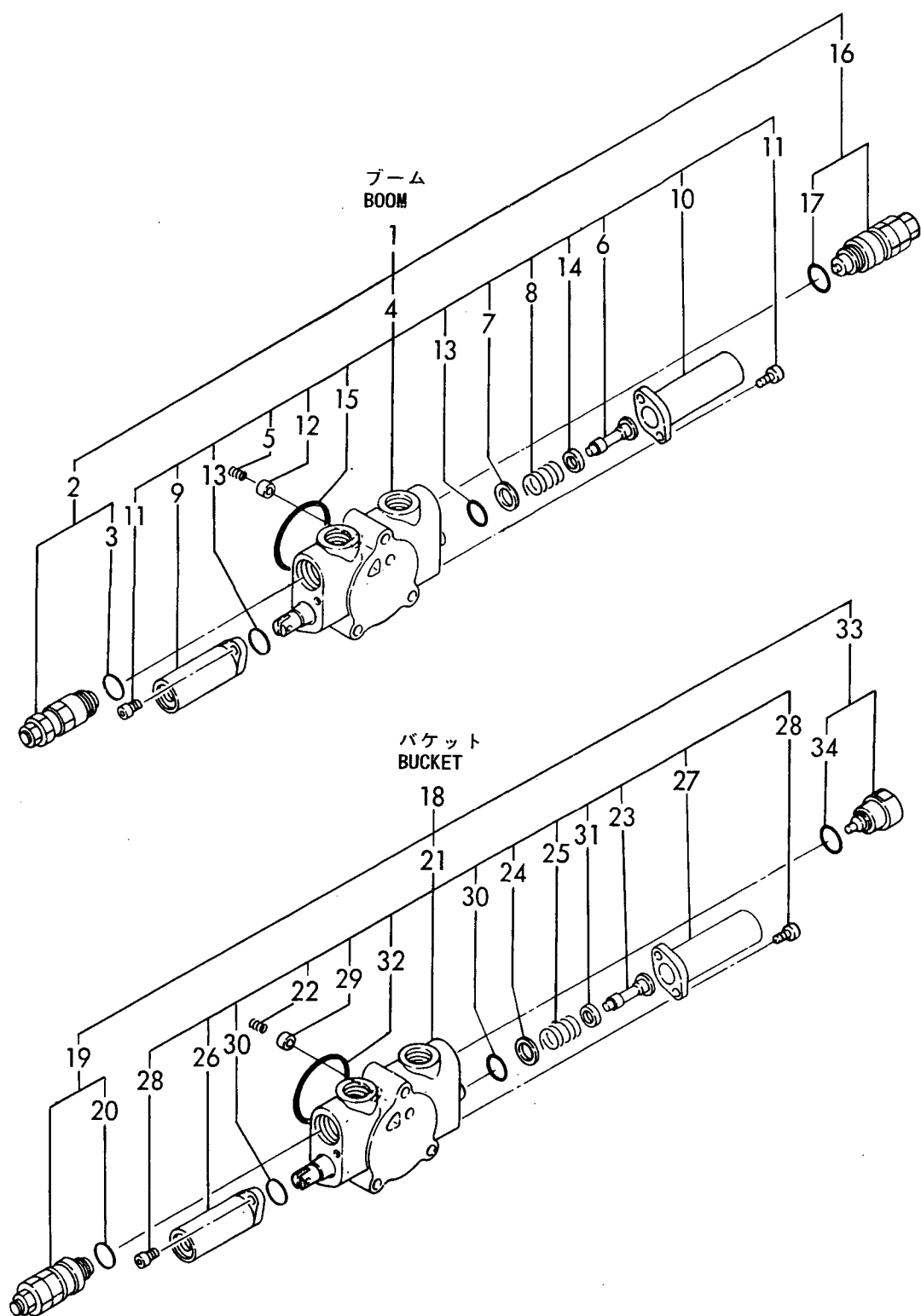
Fig. 43 コントロールバルブ(ブーム & バケット) CONTROL VALVE (BOOM & BUCKET)
