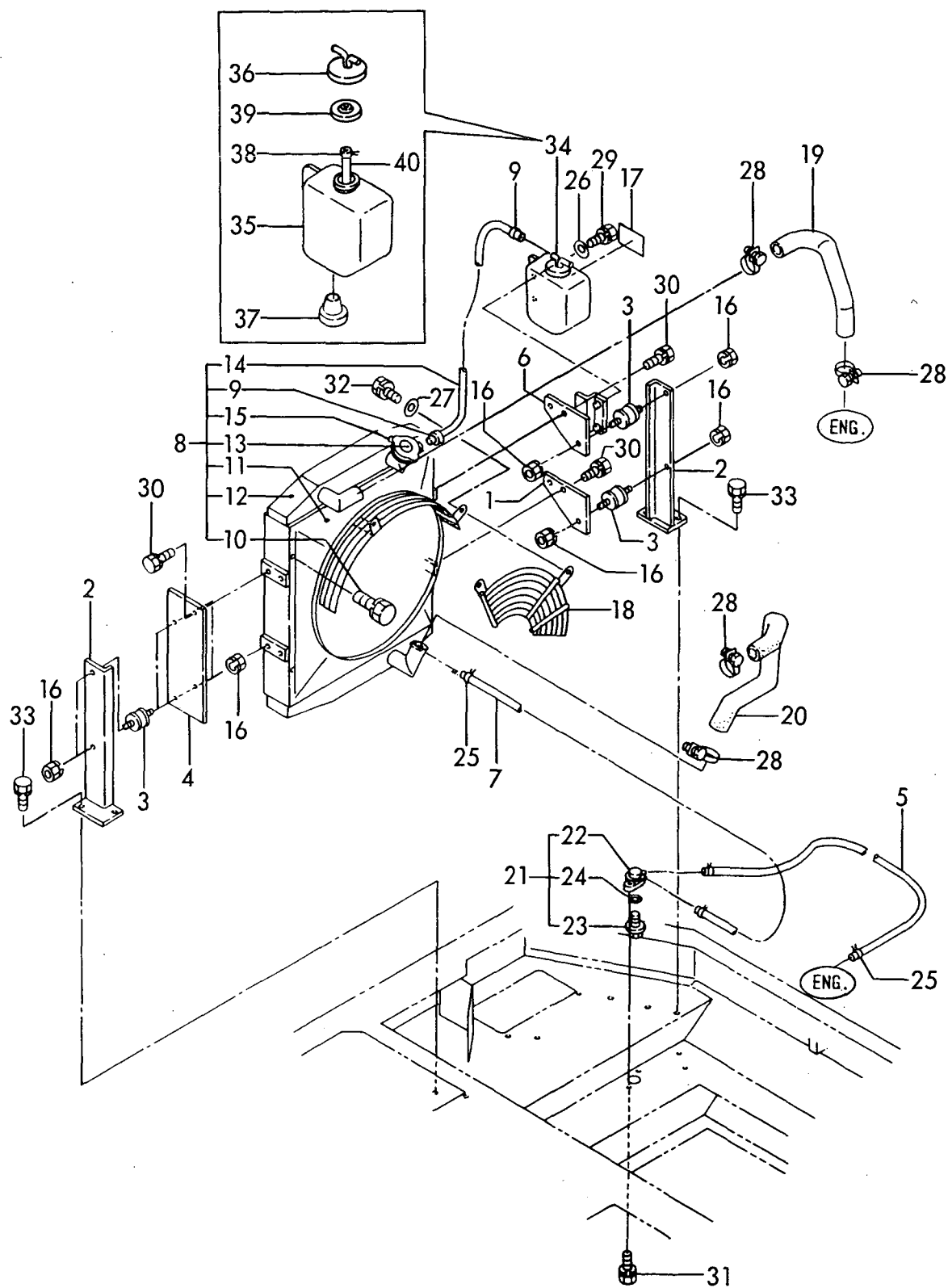
Fig. 7 ラジエータ & マウント RADIATOR & MOUNT
