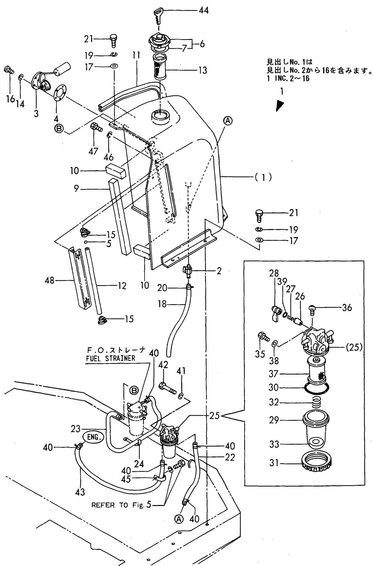
Fig. 8 F0タンク & F0パイプ FUEL TANK & FUEL LINE
