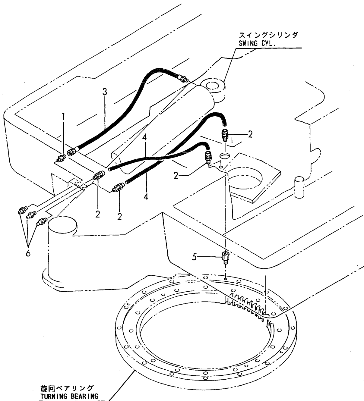
Fig. 60 遠隔グリーシング GREASING
