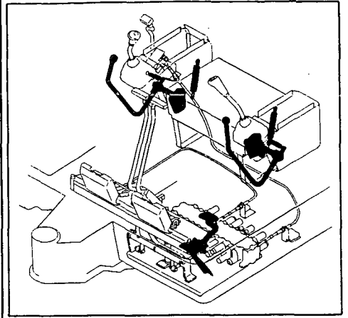
Fig. 20 操縦装置(カットオフレバー & ペダル) CONTROL EQUIPMENT(CUT-OFF LEVER & LOW-HIGH PEDAL)
