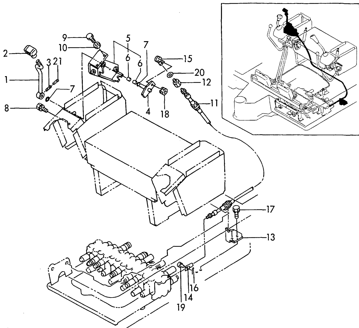
Fig. 19 操縦装置(ブレード) CONTROL EQUIPMENT (BLADE)
