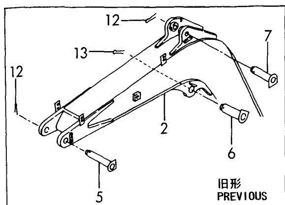
Fig. 61 61 ブーム & ブームブラケット BOOM & BOOM BRACKET
