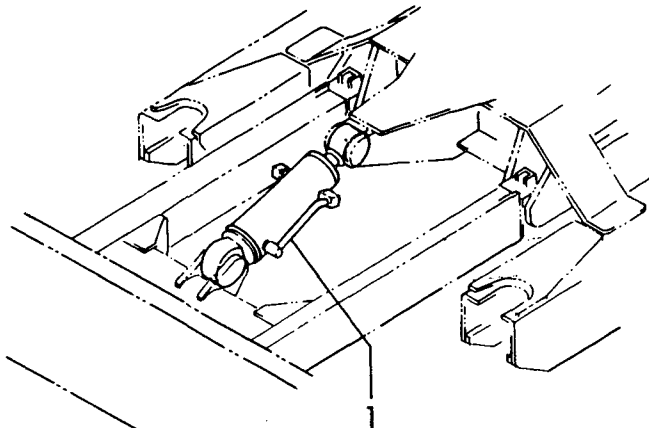
Fig. 36 ブレードシリンダ BLADE CYLINDER
