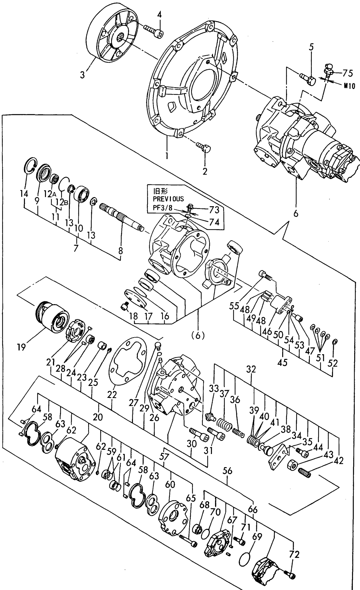
Fig. 31 ポンプ & 軸継手 HYD. OIL PUMP & JOINT
