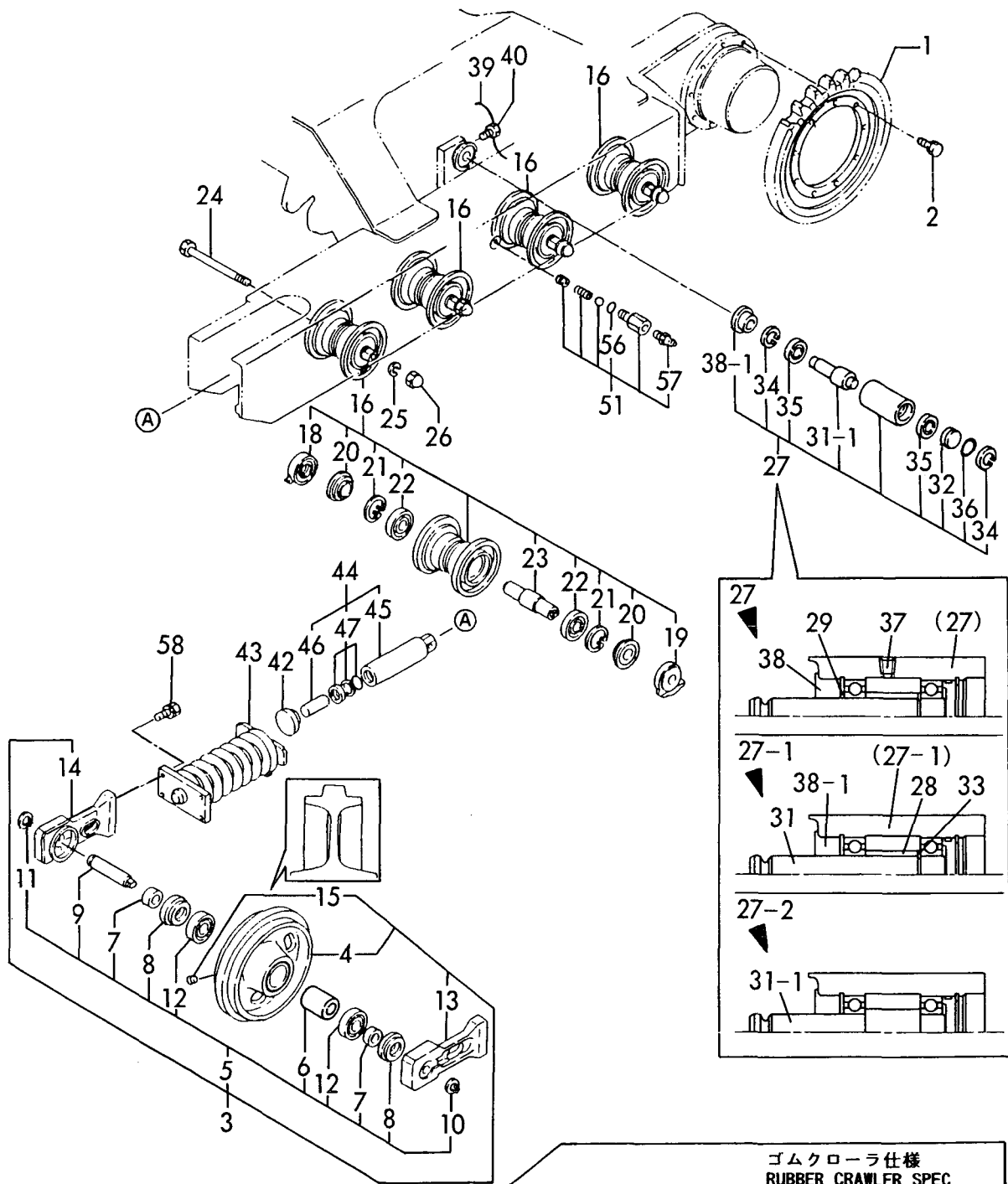
Fig. 14 ローラ & アジャスト ROLLER & ADJUST
