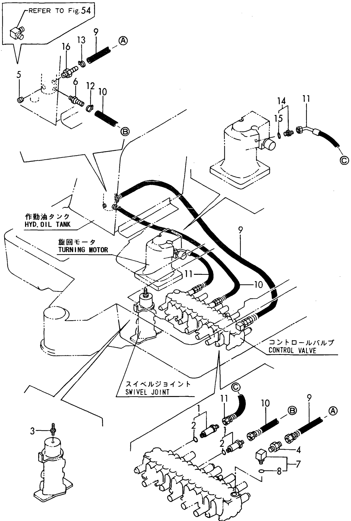
Fig. 53 油圧配管(リターン) HYD. OIL PIPING(RETURN)
