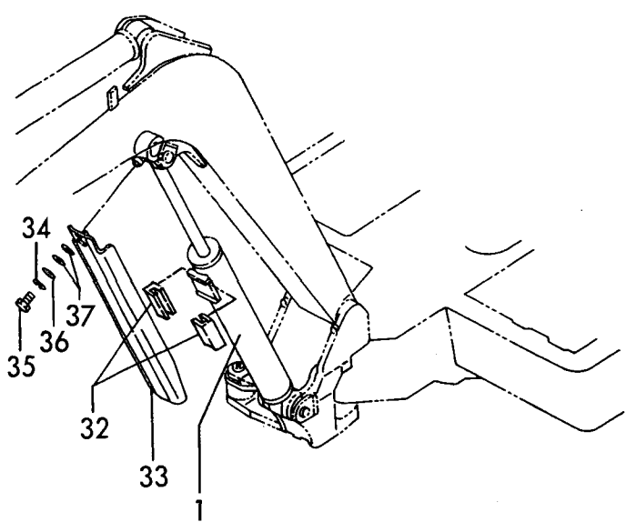
Fig. 32 ブームシリンダ BOOM CYLINDER
