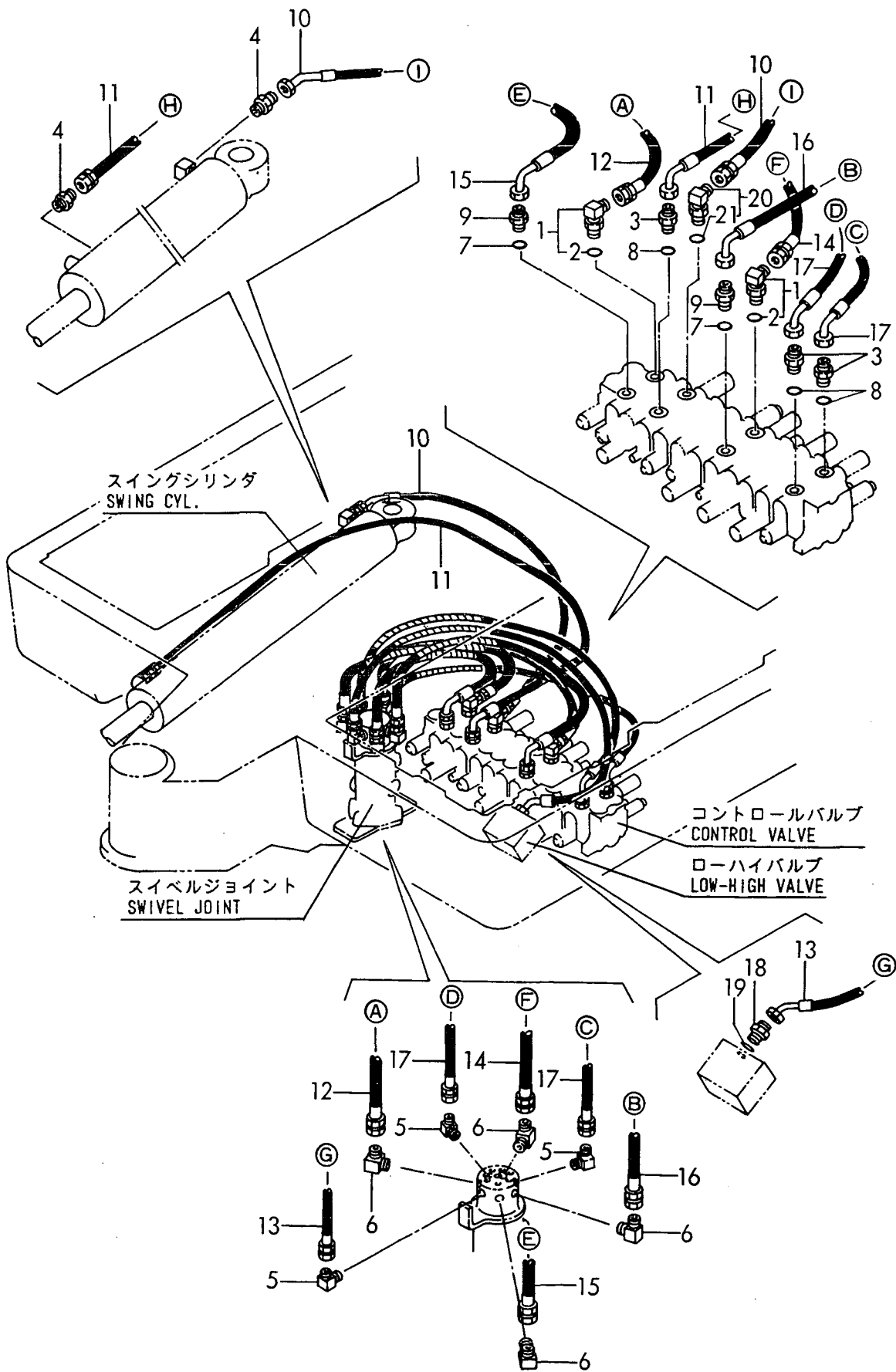
Fig. 52 油圧配管(バルブ ~スイベル, スイグ) HYD. OIL PIPING (VALVE ~ SWIVEL, SWING)
