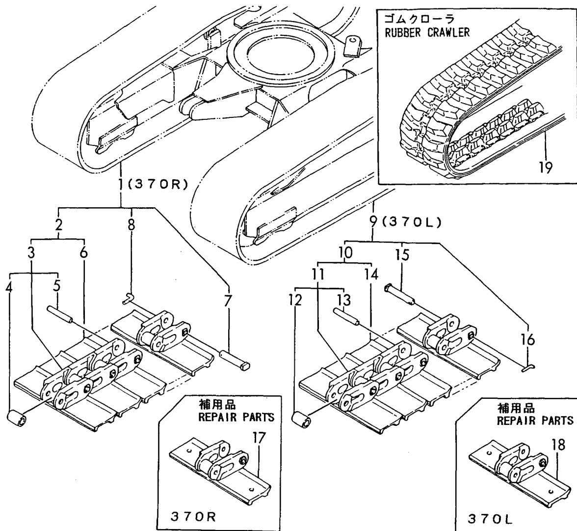
Fig. 15 クローラ CRAWLER
