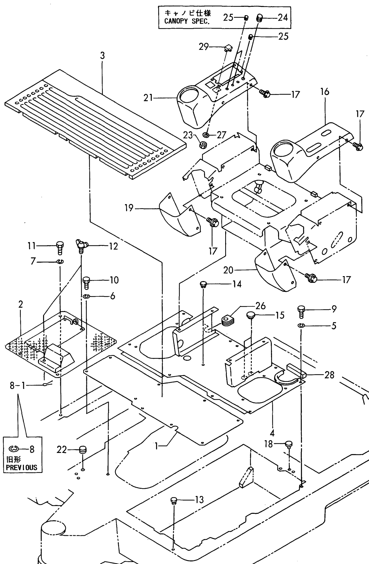
Fig. 24 ステップ & インパネ STEP & INSTRUMENT PANEL
