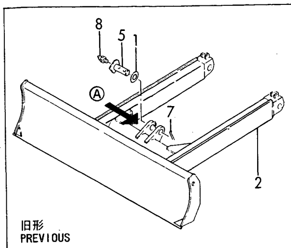
Fig. 63 ブレード BLADE
