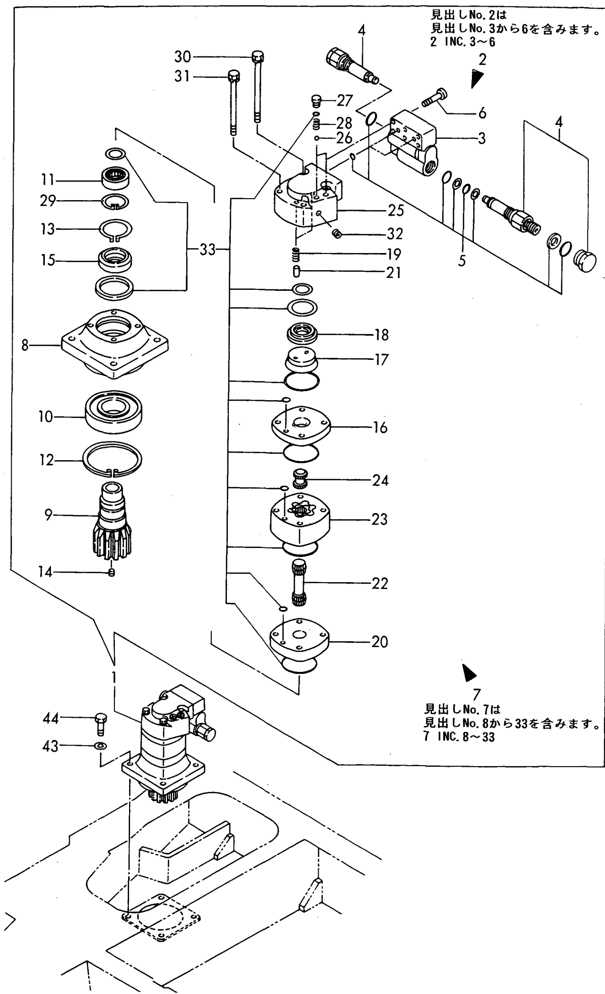
Fig. 38 回転モータ TURNING MOTOR
