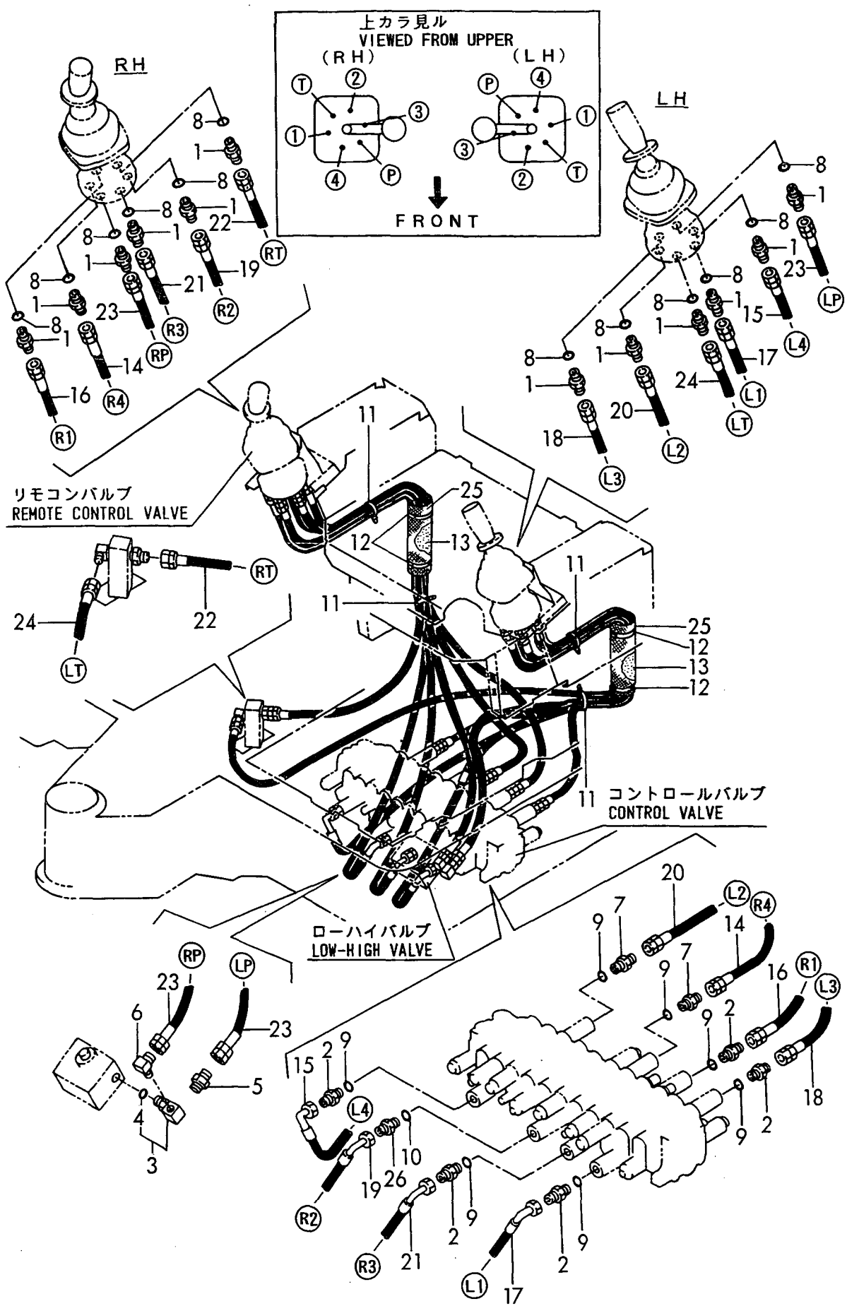
Fig. 59 コントロール配管 CONTROL PIPING
