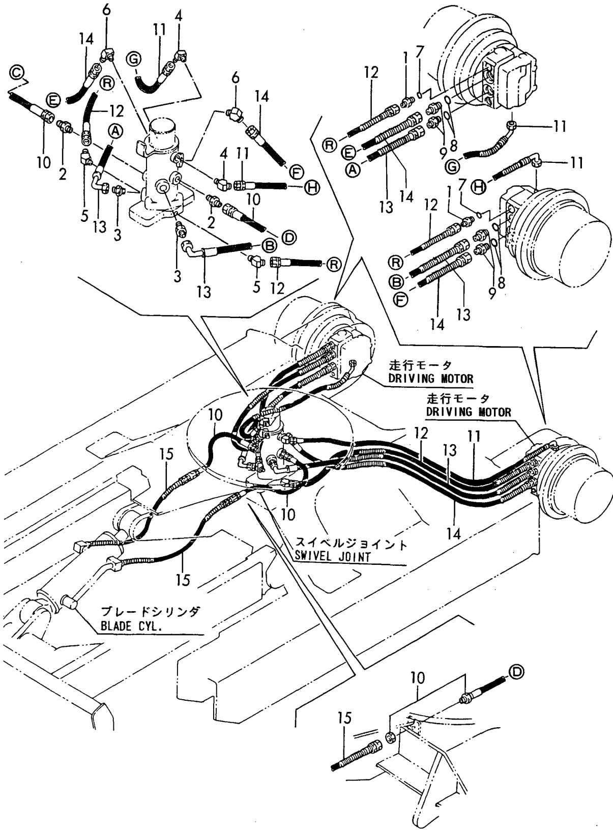
Fig. 55 油圧配管(トラックフレーム) HYD. OIL PIPING (TRACK FRAME)
